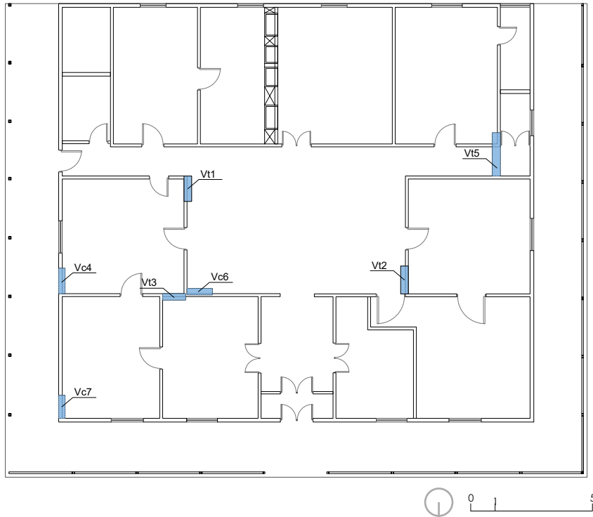
Img. n° 39 Esquema planimétrico ubicación de ventanilla tabique. © Corsa Arquitectos
