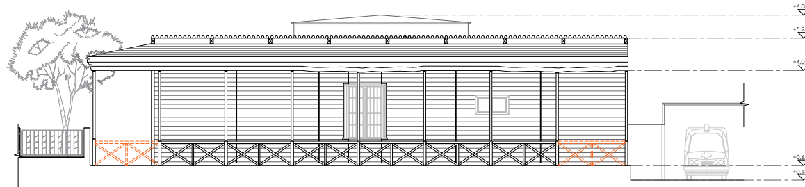
Img. n° 46 Alzado Fachada Poniente
