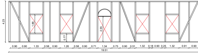
Img. n°54 Alzado Tabiquería Eje A
