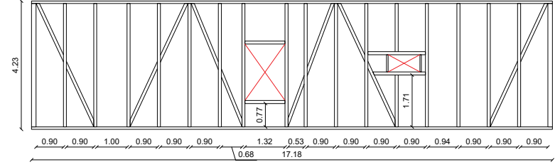
Img. n°55 Alzado Tabiquería Eje 14
