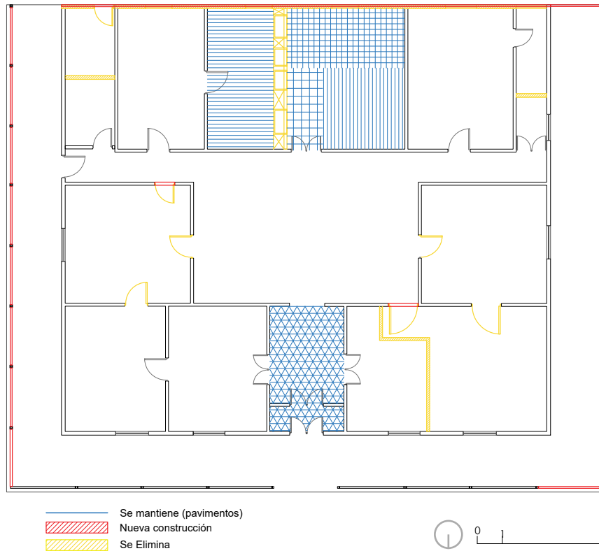
Img. n°8o Planta propuesta de intervención en el inmueble.
