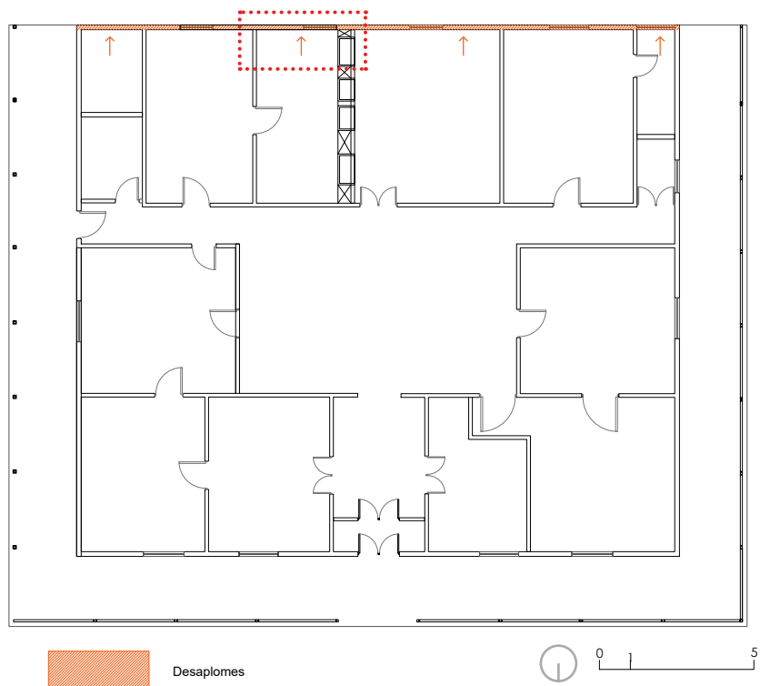
Img. n°66 Planta de ubicación de catastro de desaplome relacionados a los propios asentamientos detectados in situ. © Corsa Arquitectos.
