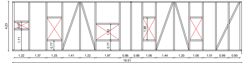
Img. n°56 Alzado Tabiquería Eje E
