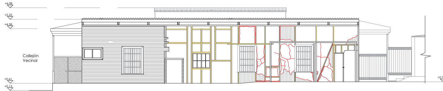
Img. n°60 Alzado Sur levantamiento catastro de grietas. © Corsa Arquitectos.
