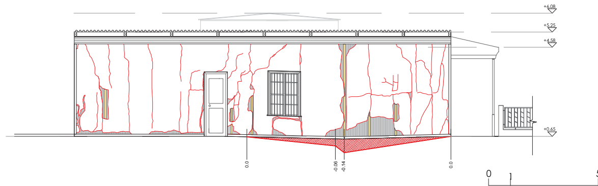
Img. n° 61 Alzado Lateral Oriente son corredor levantamiento catastro de grietas y desaplome. © Corsa Arquitectos.
