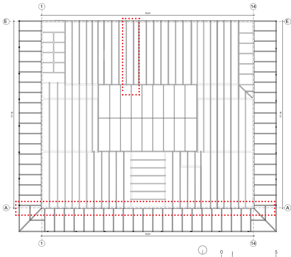
Img n° 68 Planta de cielo constatación de humedades. © Corsa Arquitectos.
