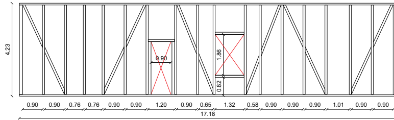
Img. n°53 Alzado Tabiquería Eje 1
