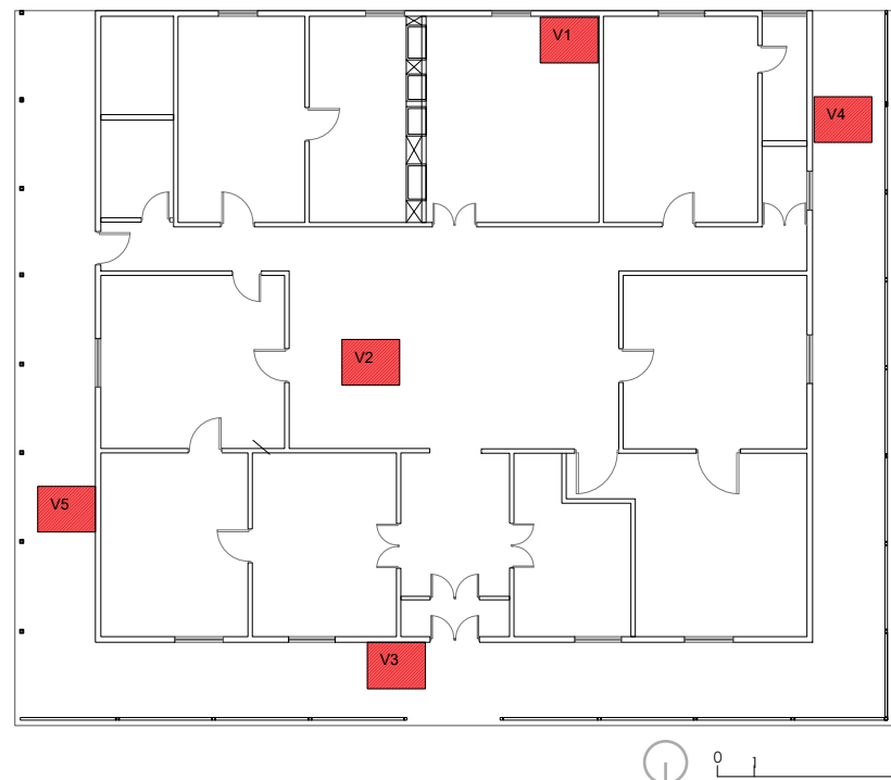
Img. n° 34 Esquema planimétrico ubicación de ventanilla subsuelo. © Corsa Arquitectos
